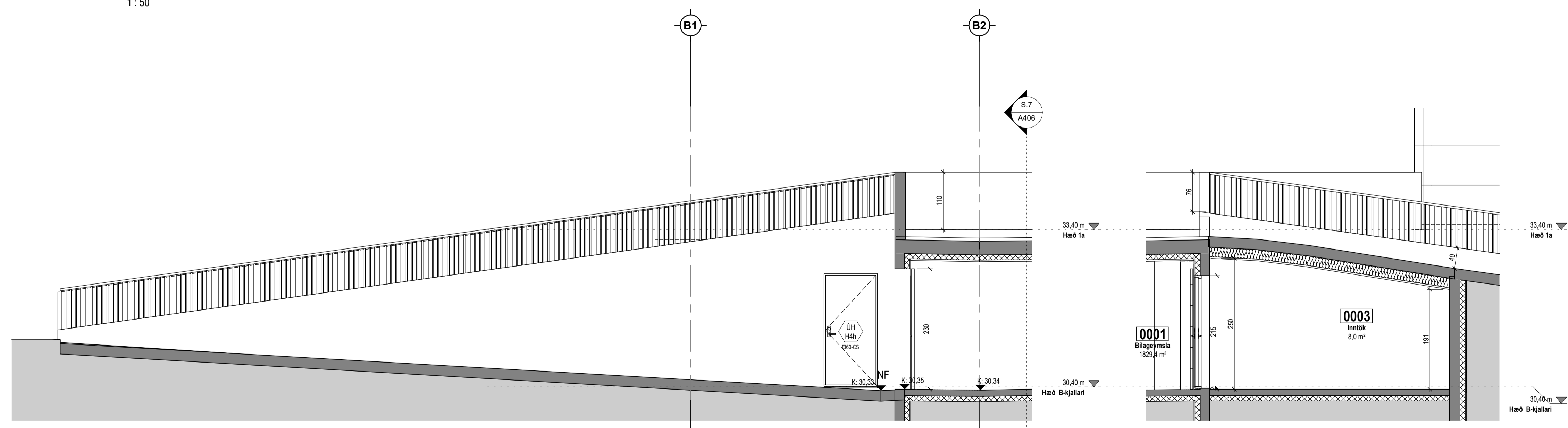
SU-Snið 4 1:50
