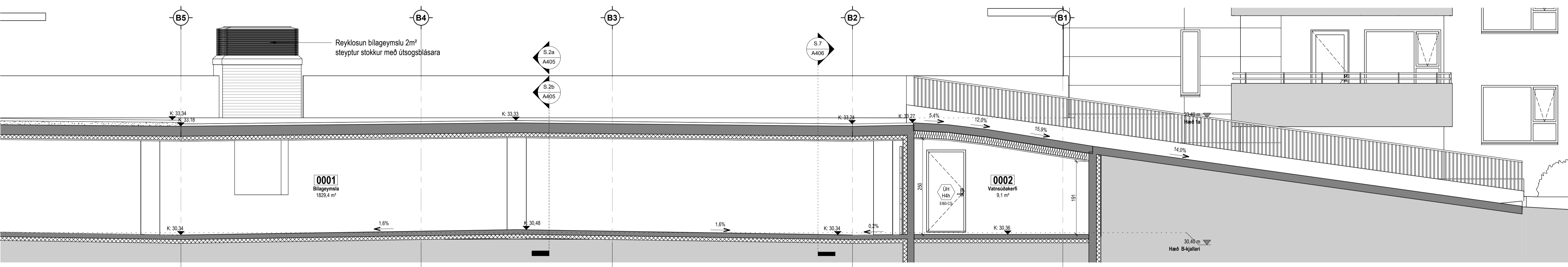
SU-Snið 4 1:50
